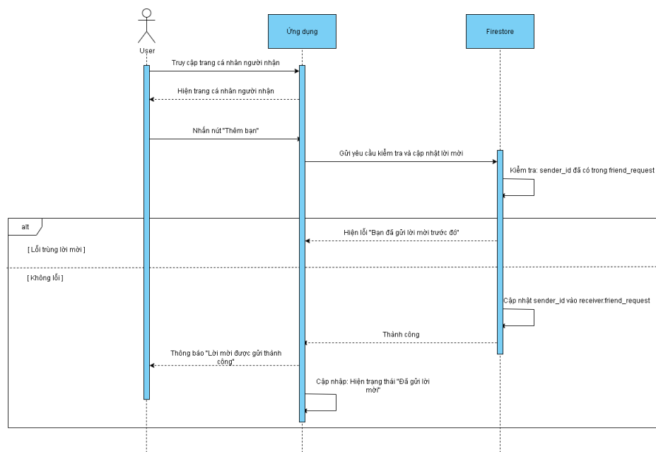
Hình 20: Sequence Diagram: Gửi lời mời kết bạn
