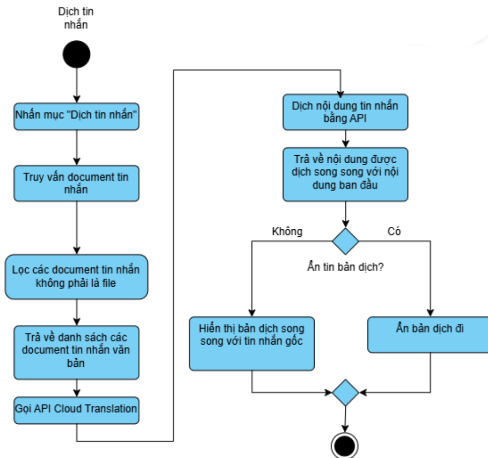
Hình 12: Activity Diagram: Quy trình Dịch tin nhắn
