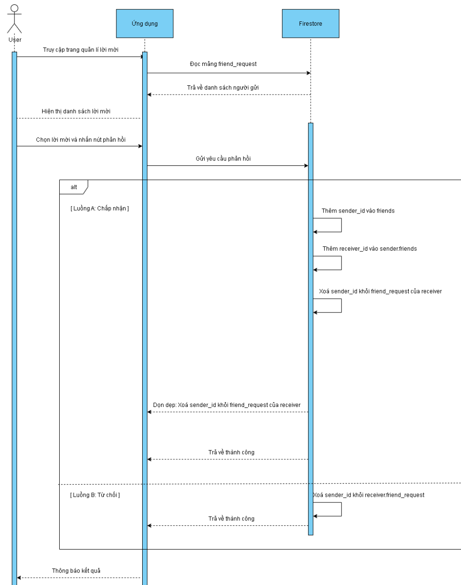
Hình 21: Sequence Diagram: Phản hồi lời mời kết bạn
