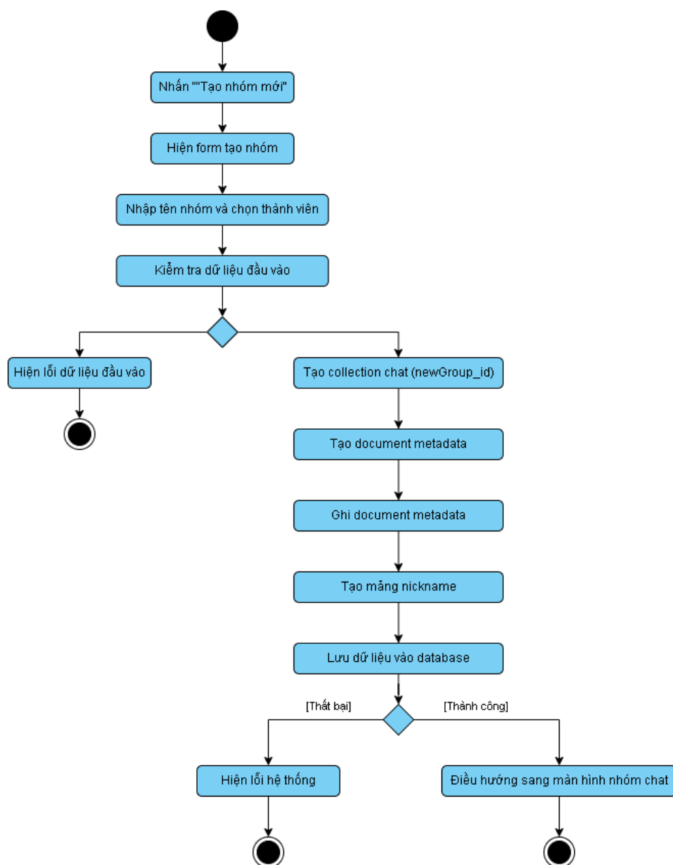
Hình 9: Activity Diagram: Quy trình Tạo nhóm chat
