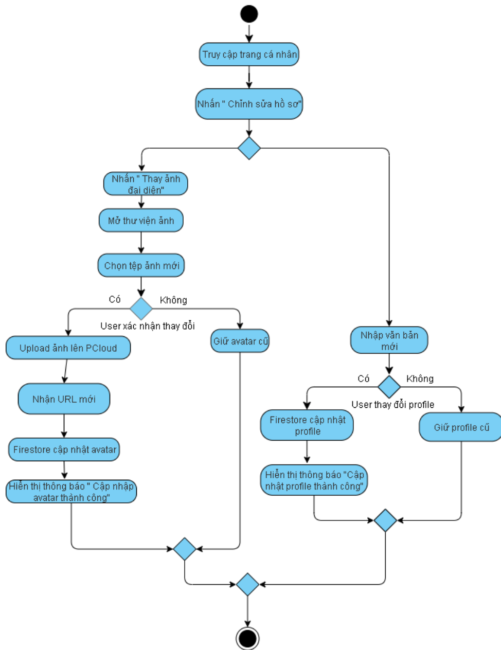
Hình 13: Activity Diagram: Quy trình Chỉnh sửa hồ sơ
