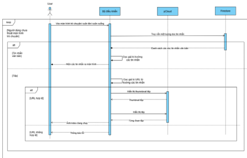
Hình 25: Sequence Diagram: Hiện thị lịch sử
