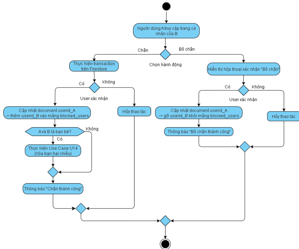
Hình 15: Activity Diagram: Quy trình Chặn và Bỏ chặn
