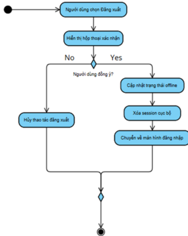
Hình 4: Activity Diagram: Quy trình Đăng xuất
