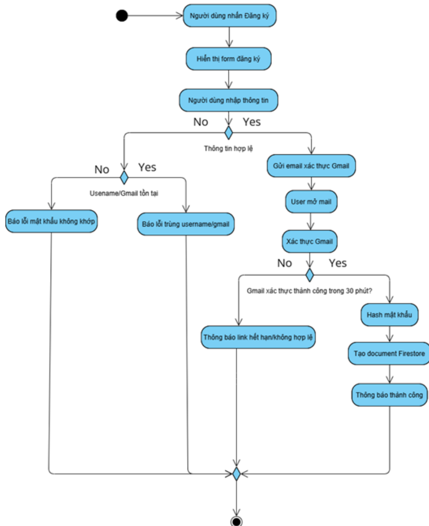
Hình 2: Activity Diagram: Quy trình Đăng ký tài khoản
