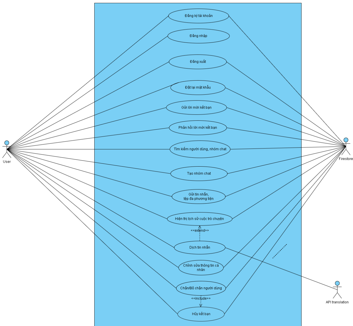
Hình 1: Sơ đồ Use-case tổng quát của hệ thống TransChat ( Xem ảnh gốc tại đây )
