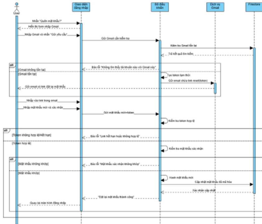
Hình 19: Sequence Diagram: Đặt lại mật khẩu
