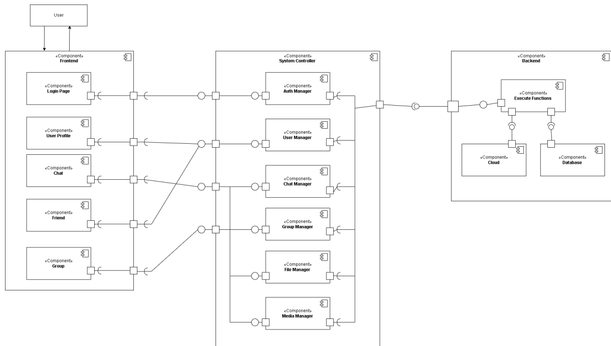
Hình 33: Component Diagram ( Xem ảnh gốc tại đây )
