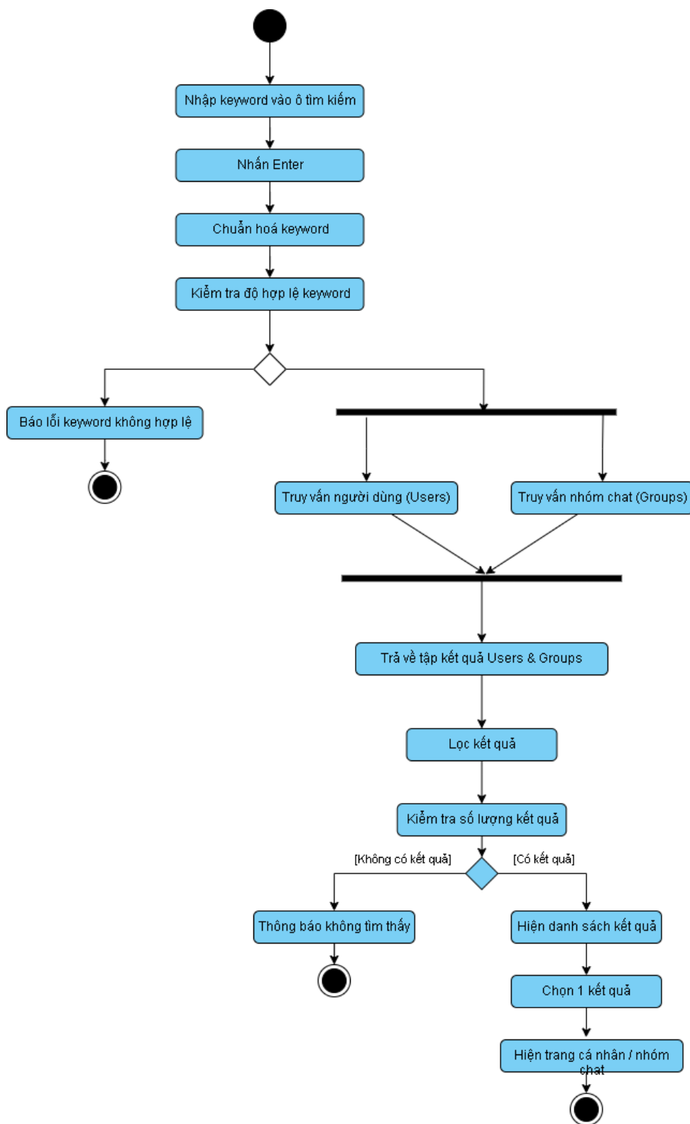
Hình 8: Activity Diagram: Quy trình Tìm kiếm
