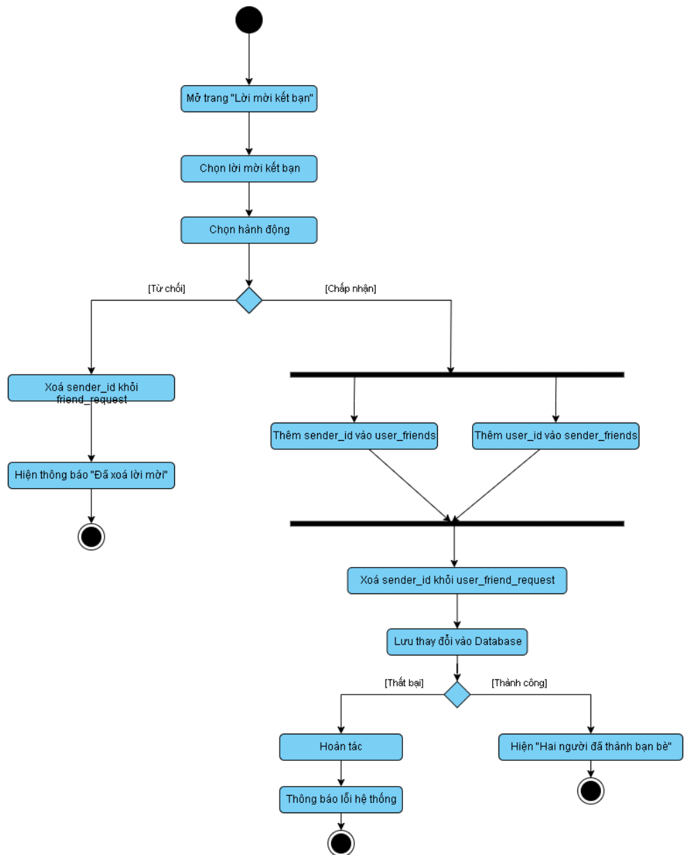
Hình 7: Activity Diagram: Quy trình Phản hồi kết bạn
