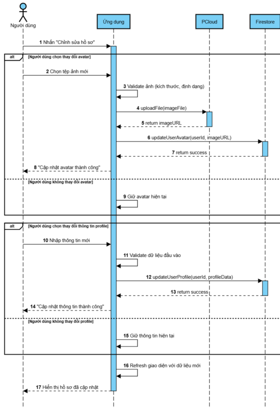
Hình 27: Sequence Diagram: Chỉnh sửa hồ sơ
