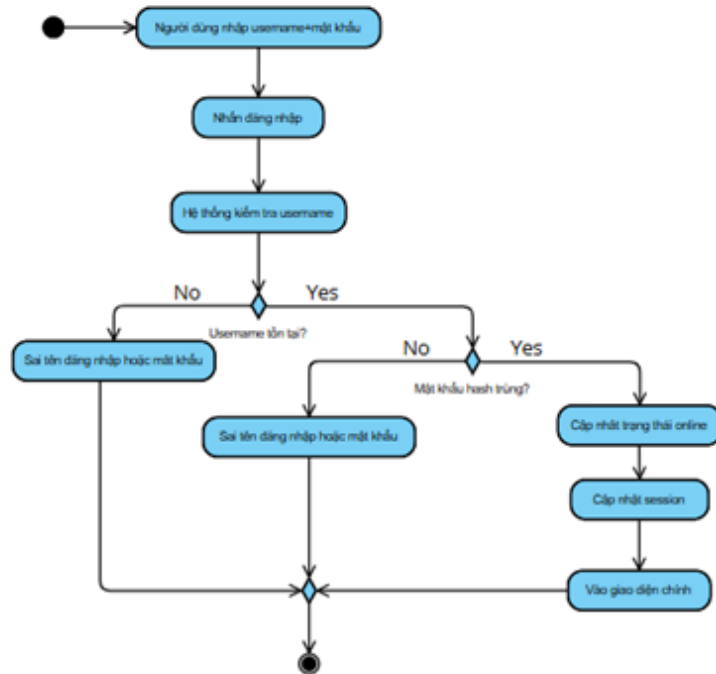
Hình 3: Activity Diagram: Quy trình Đăng nhập
