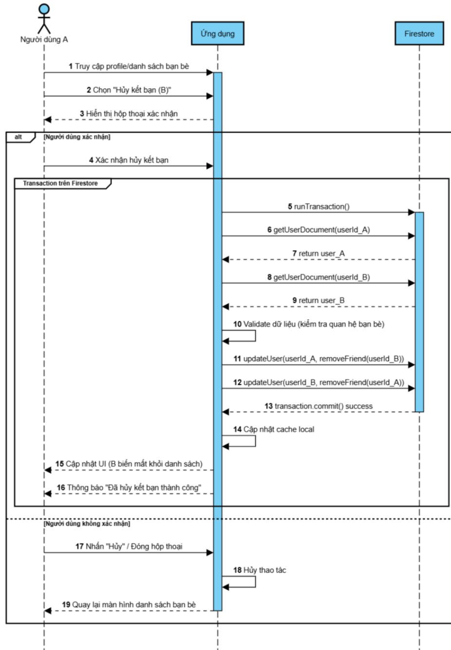
Hình 28: Sequence Diagram: Hủy kết bạn
