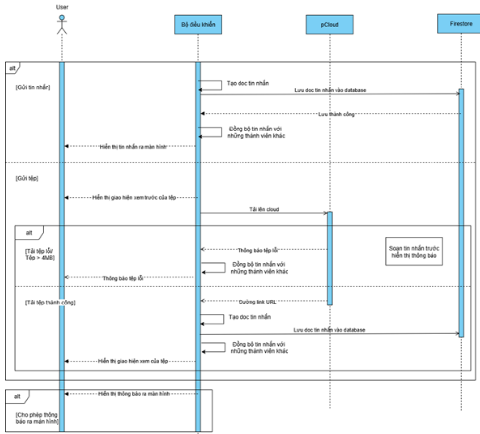
Hình 24: Sequence Diagram: Gửi tin nhắn
