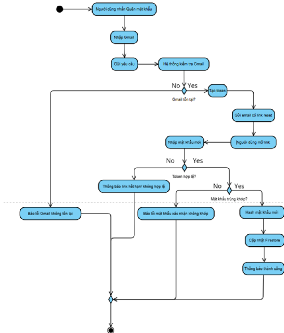
Hình 5: Activity Diagram: Quy trình Đặt lại mật khẩu
