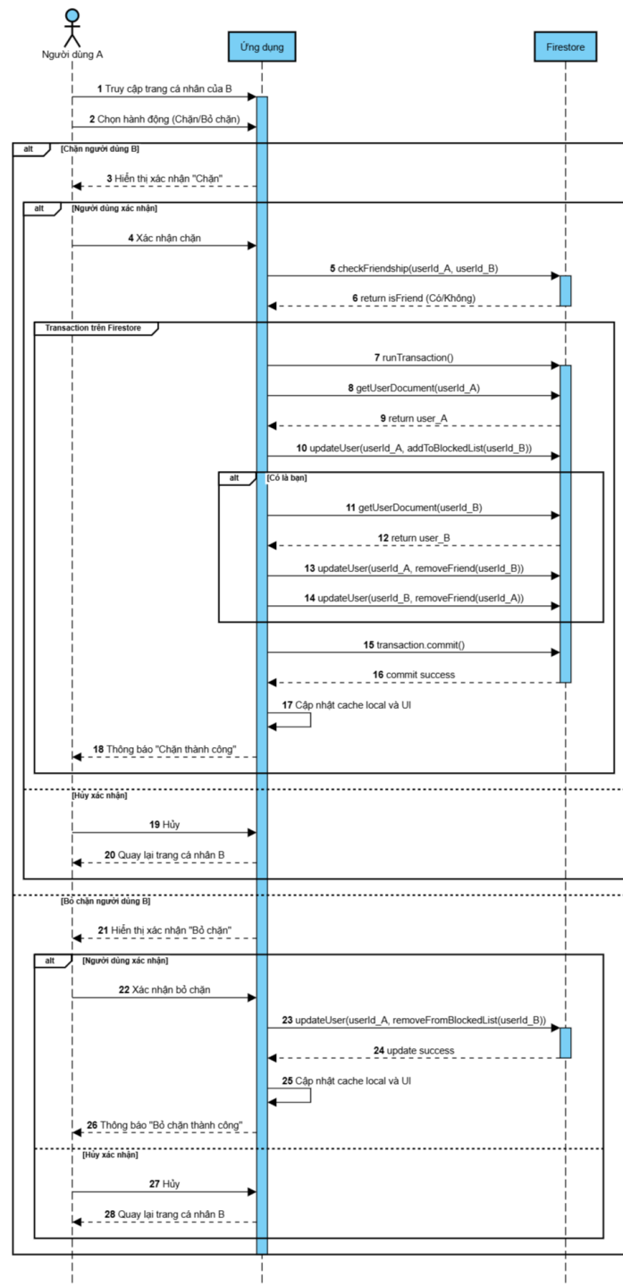
Hình 29: Sequence Diagram: Chặn và Bỏ chặn
